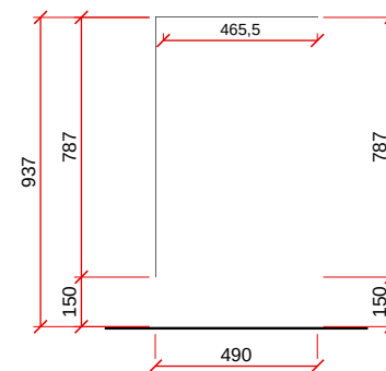
VISTA C - ESC. 1:25
